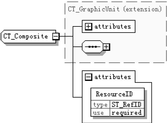
图 71 复合对象基本结构
