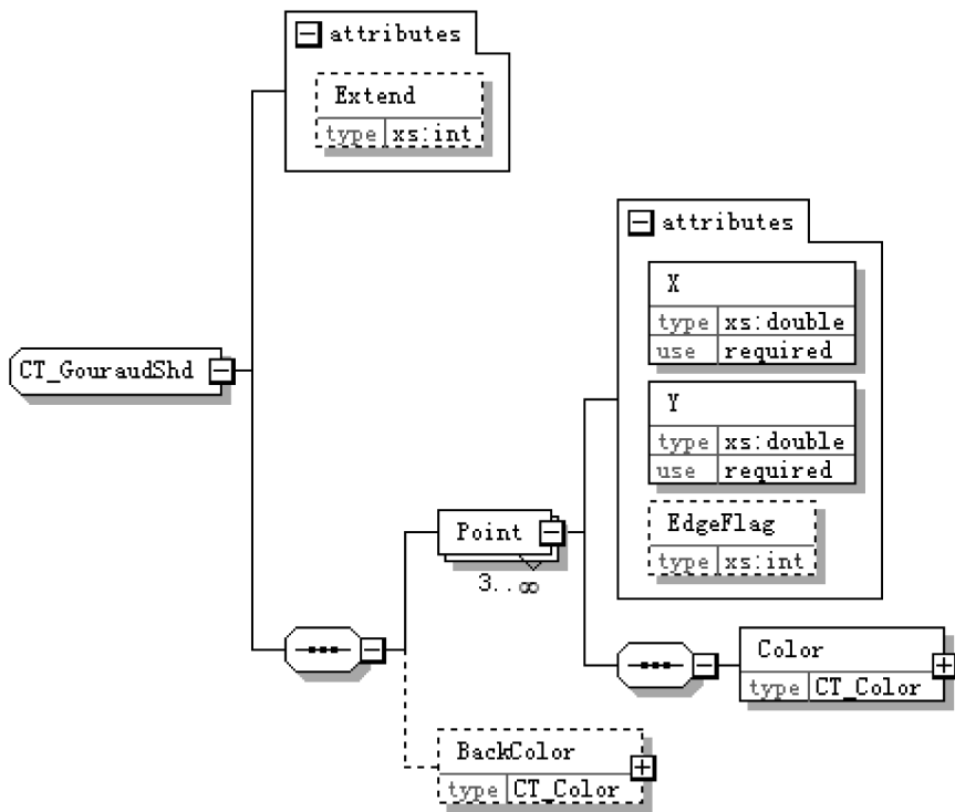
图 41 高洛德渐变结构
