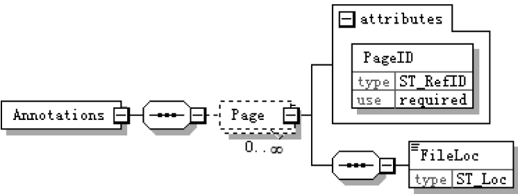
图 80 注释列表结构
